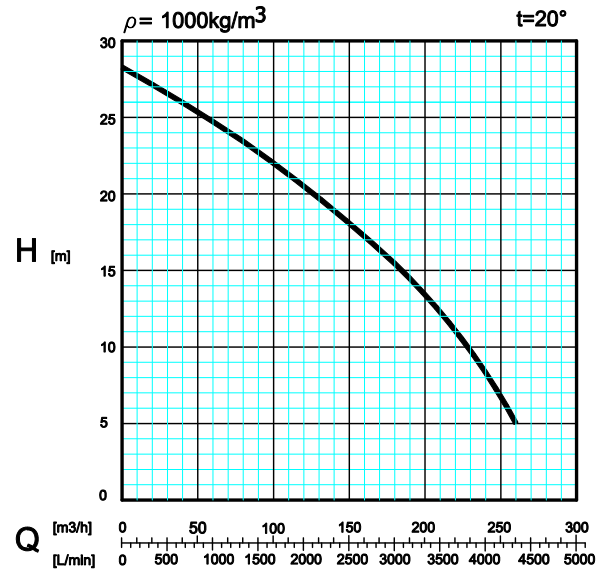
Charakterystyka pracy pompy
