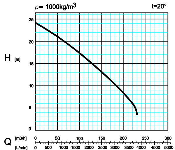
Charakterystyka pracy pompy
