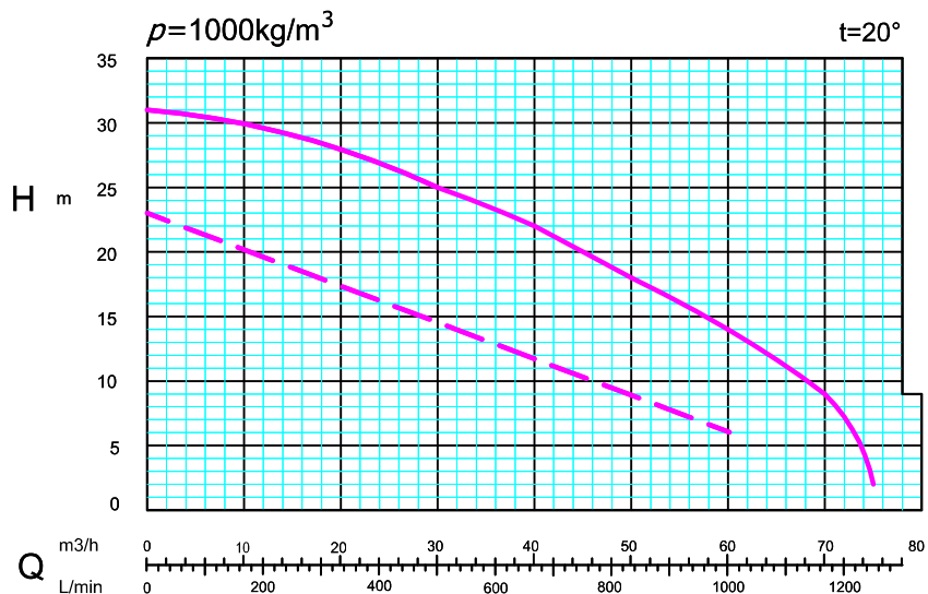
Характеристики погружного насоса
