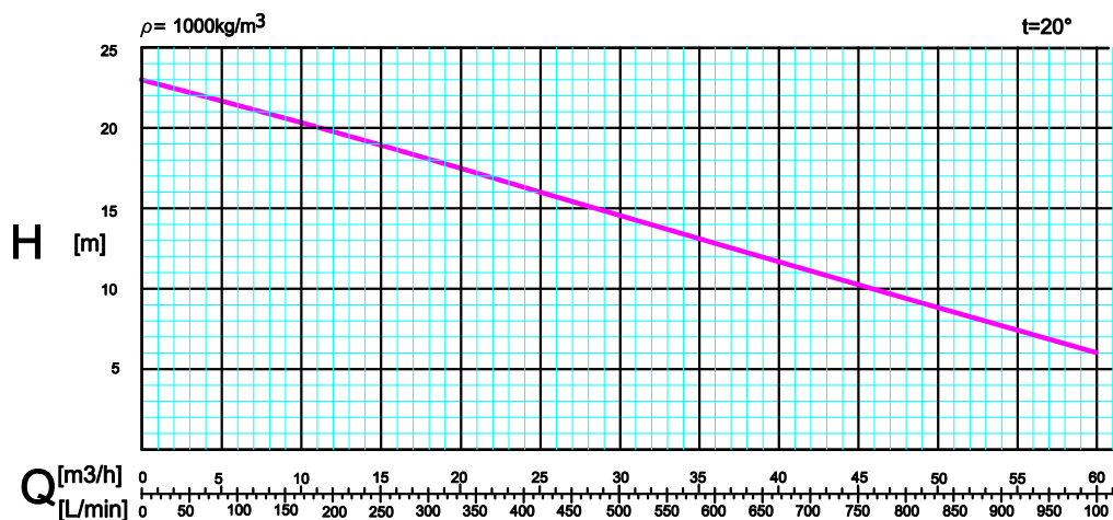
Charakterystyka pracy pompy
