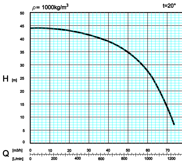
Charakterystyka pracy pompy
