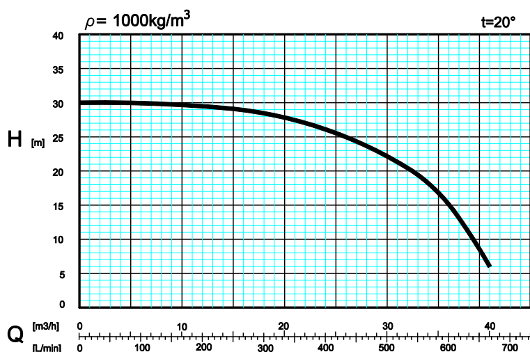
Charakterystyka pracy pompy
