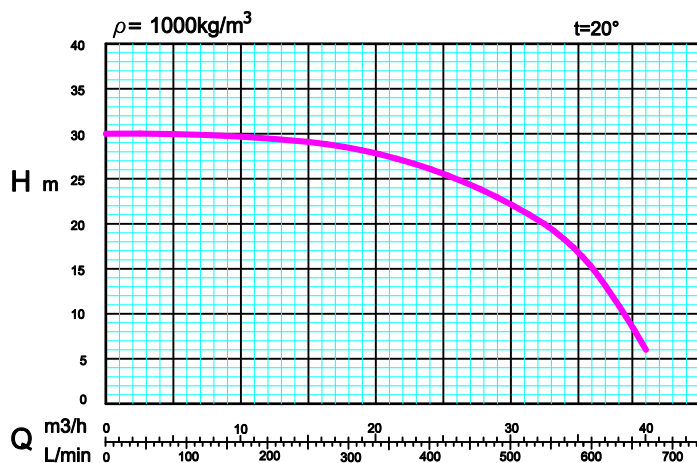
Charakterystyka pracy pompy
