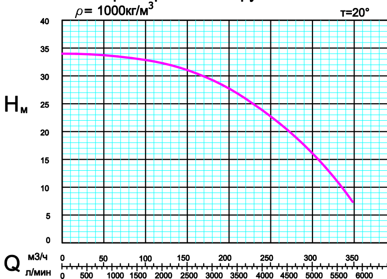
Характеристики погружного насоса
